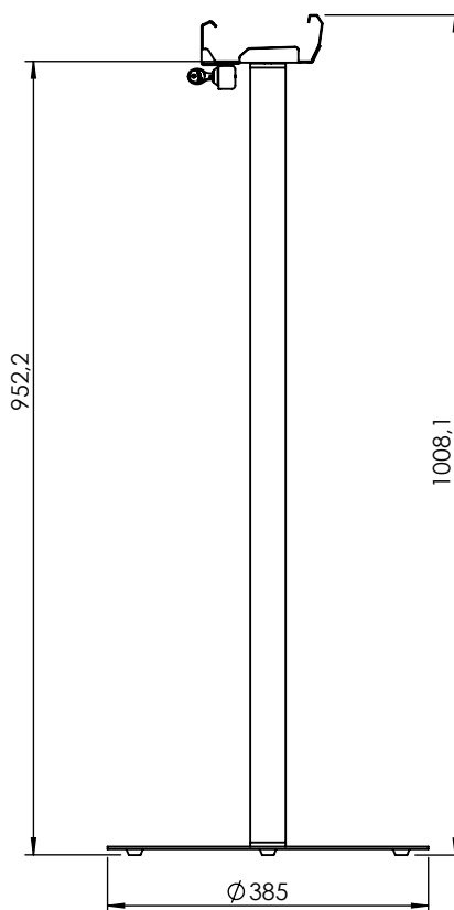
Edelstahlsäule | Abmessungen in mm
